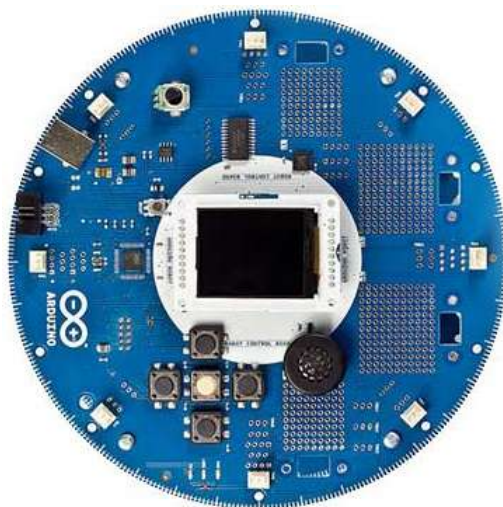
Obrázek 2.12: Arduino Robot
