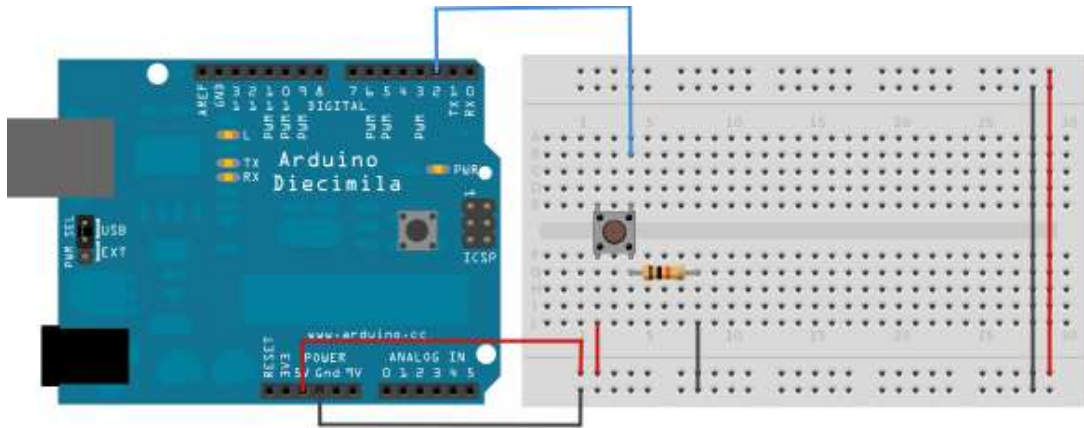
Obrázek 13.1: Tlačítko - INPUT
