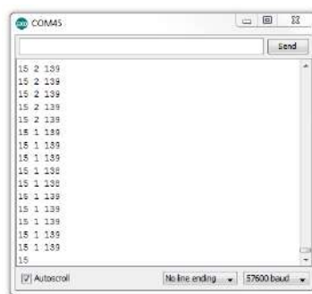
Obrázek 44.2: Monitor sériové linky
