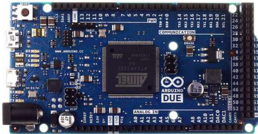
Obrázek 2.10: Arduino Due
