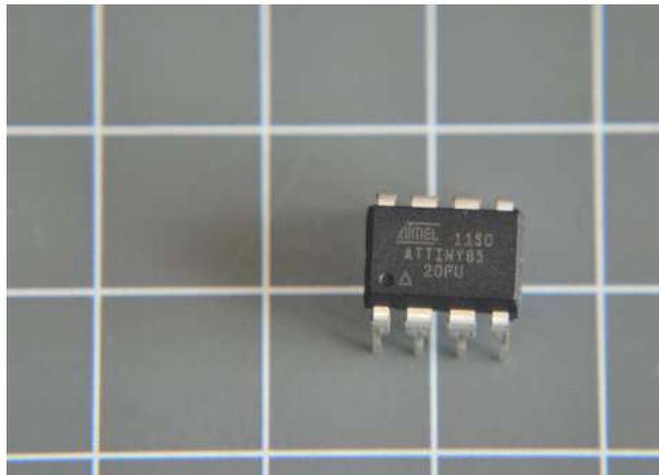
Obrázek 60.2: ATtiny 85
