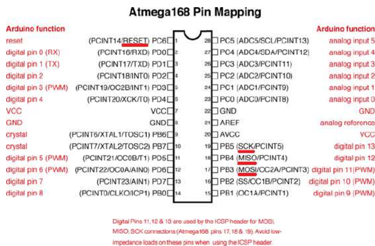
Obrázek 61.2: ATmega 168 pinout
