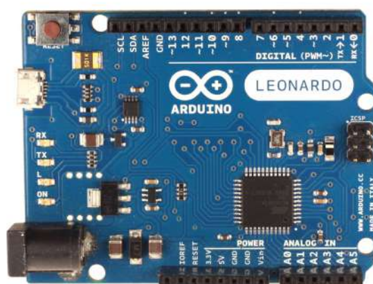
Obrázek 33.1: Arduino Leonardo
