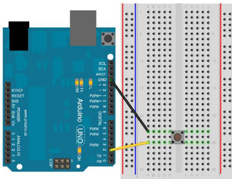
Obrázek 13.2: Tlačítko – INPUT_PULLUP
