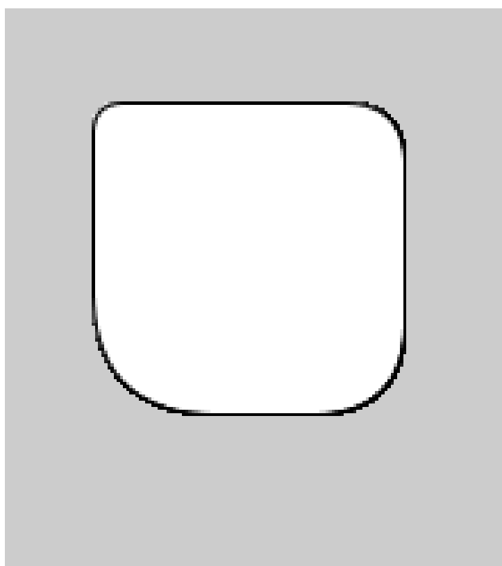
Obrázek 40.8: Funkce rect()
